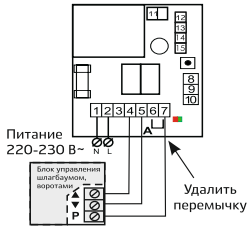
Рис. 3. Подключение к раздельным входам «ОТКРЫТ» и «ЗАКРЫТ»
