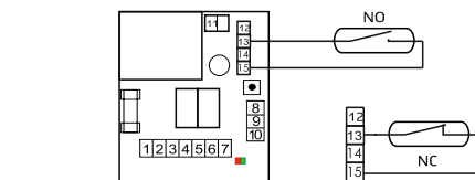
Рис. 4. Подключение геркона
