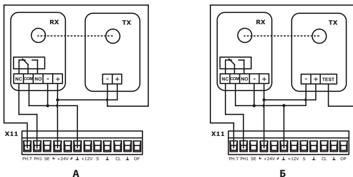
Рисунок 5. Подключение фотоэлементов при реализации автоматической проверки их работы ( Фототест ): А — фотоэлементы с типовым подключением, Б — фотоэлементы со специальным выходом TEST
