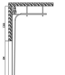
Высокий тип монтажа с верхним расположением вала
