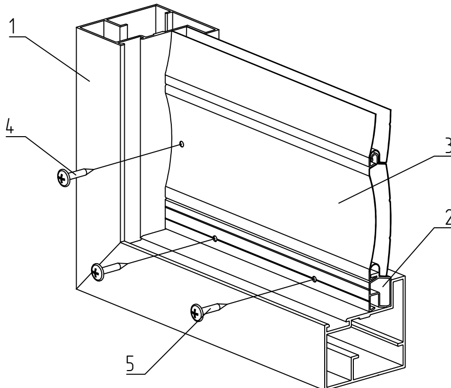
Рис. 8.32 – Установка «нижней» части заполнения: 1 – створка, 2 – профиль притвора FLGU.400.0501, 3 – профиль AG/77, 4 – винт самонарезающий 4,2x19SGX, 5 – винт самонарезающий 4,2x25SGX
