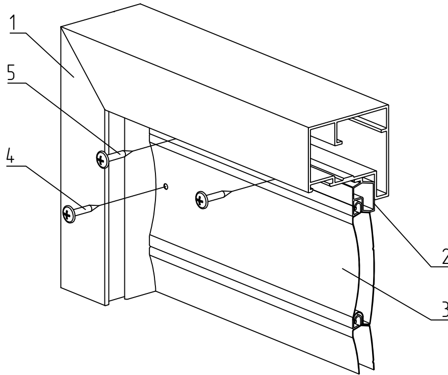
Рис. 8.31 – Установка «верхней» части заполнения: 1 – створка, 2 – профиль притвора FLGU.400.0501, 3 – профиль AG/77, 4 – винт самонарезающий 4,2x19SGX, 5 – винт самонарезающий 4,2x25SGX
