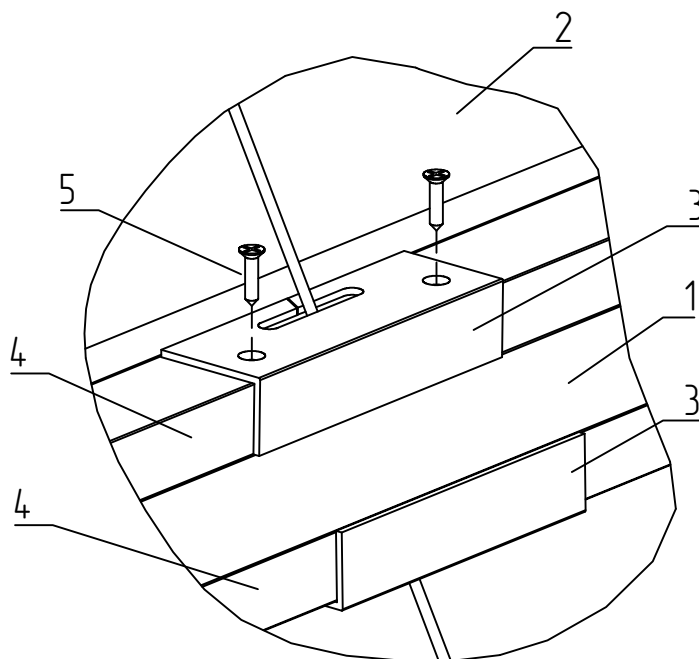
Рис. 9.6 – Установка крышки FLGU.400.0723
