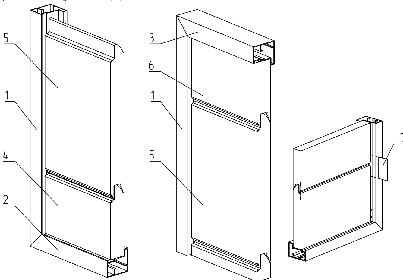
Рис. 8.25 – Установка сэндвич-панелей и подкладок
