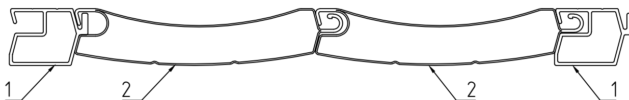
Рис. 8.29 – Заполнение AG/77: 1 – профиль притвора FLGU.400.0501, 2 – профиль AG/77
