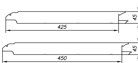
Рис. 3.4 – Сэндвич-панель Сэндвич-панель с рисунком «L-гофр»
