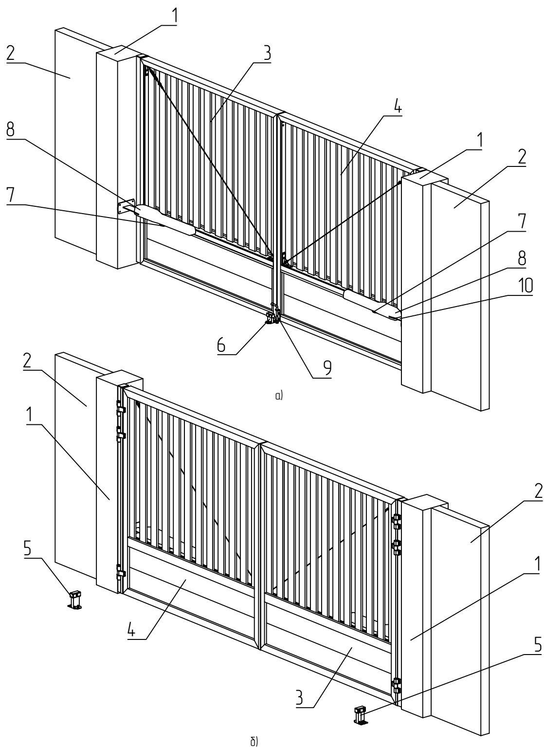
Рис. 7.4.3 – Распашные ворота со встроенным типом монтажа, открывание наружу с комбинированным заполнением – нижняя ячейка из заполнения сэндвич-панелью, верхняя из заполнения «широким» профилем:
