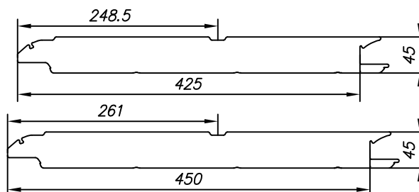
Рис. 3.3 – Сэндвич-панель с рисунком «М-гофр»
