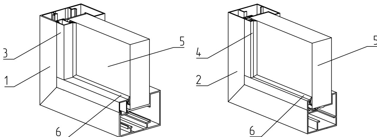
Рис. 9.2 – Установка штапика FLGU.400.0301, FLGU.400.0303 и уплотнителя FRK12 в раму с заполнением из сэндвич-панелей.
