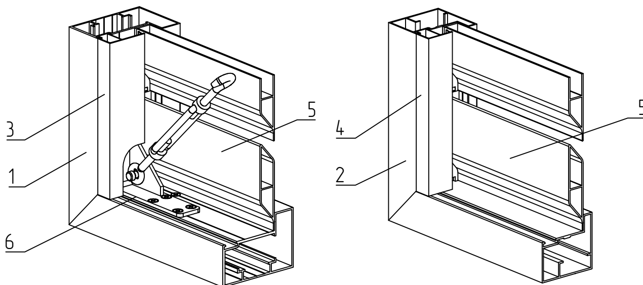
Рис. 9.4 – Установка штапика FLGU.400.0302, FLGU.400.0304 и уплотнителя FRK12 в раму с заполнением из алюминиевых профилей "жалюзи".
