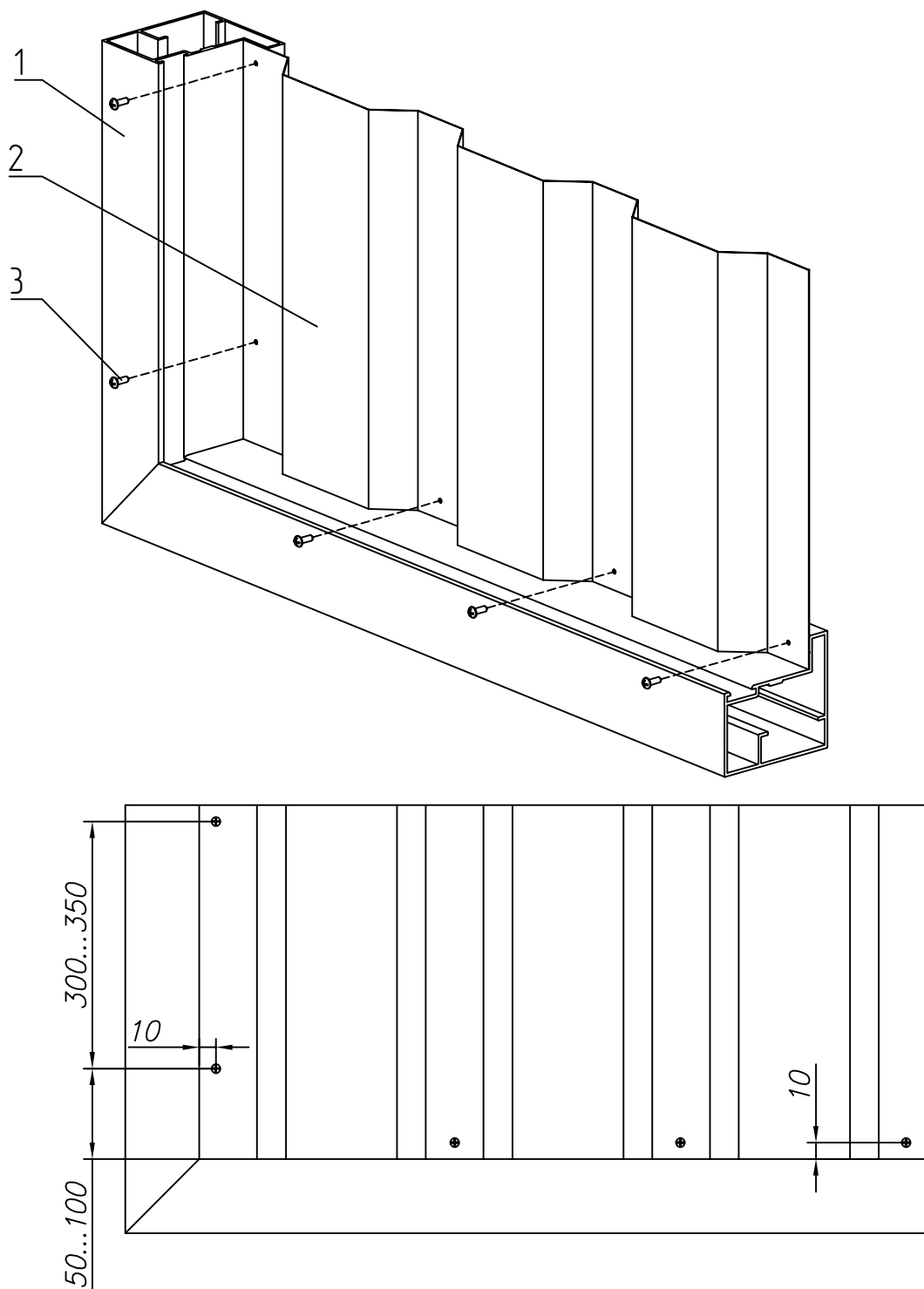
Рис. 8.33 – Установка заполнения из профилированного листа со встроеным типом монтажа:
