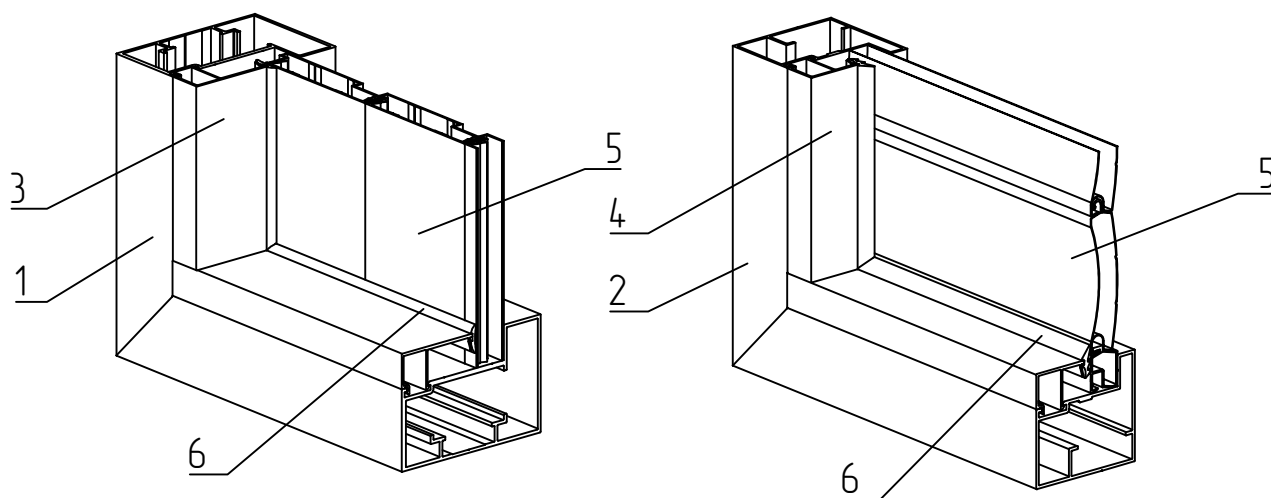
Рис. 9.3 – Установка штапика FLGU.400.0302, FLGU.400.0304 и уплотнителя FRK39 в раму с заполнением из сплошного алюминиевого профиля, профиля AG/77, PD/77.
