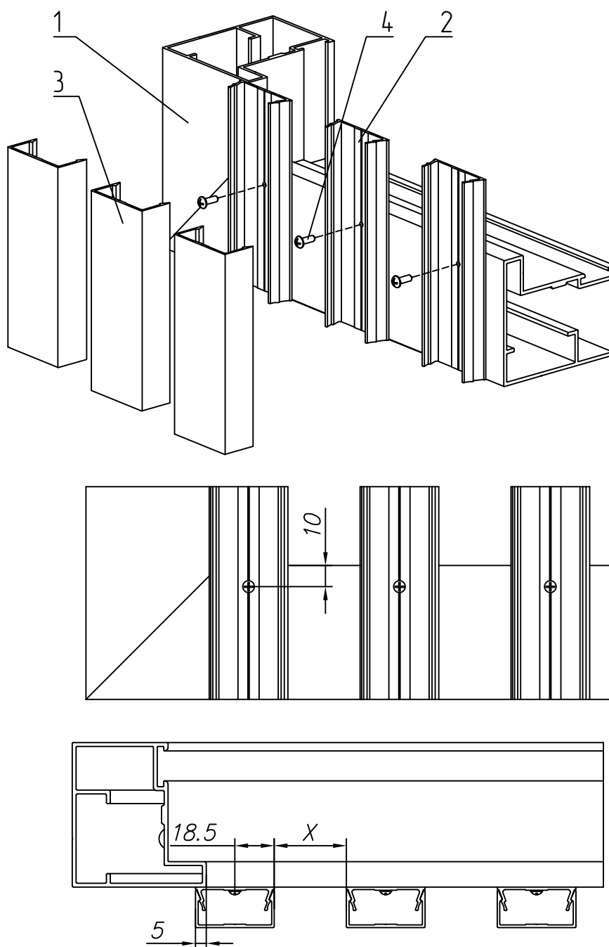
Рис. 8.7 – Монтаж заполнения с накладным типом монтажа из профилей разреженного заполнения шириной 37 мм:
