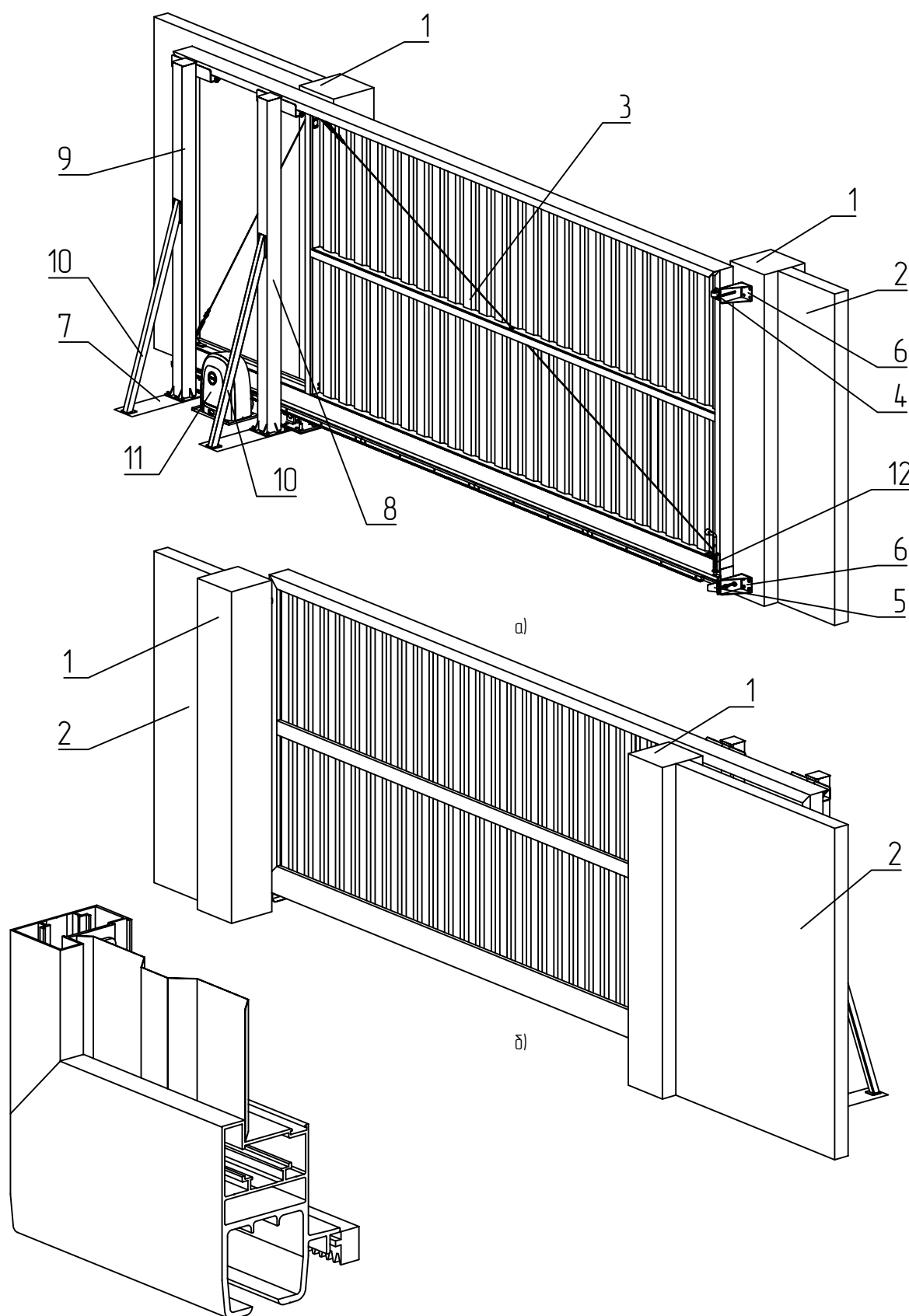
Рис. 7.18 – Откатные самонесущие ворота с вертикальным встроенным заполнением профилированным листом, открывание влево:
