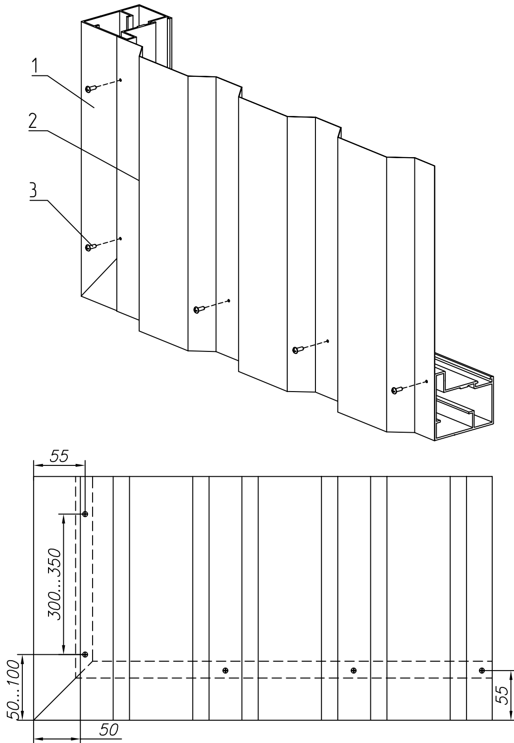
Рис. 8.34 – Установка заполнения из профилированного листа с накладным типом монтажа: 1 – створка, 2 – лист профилированный, 3 – крепеж
