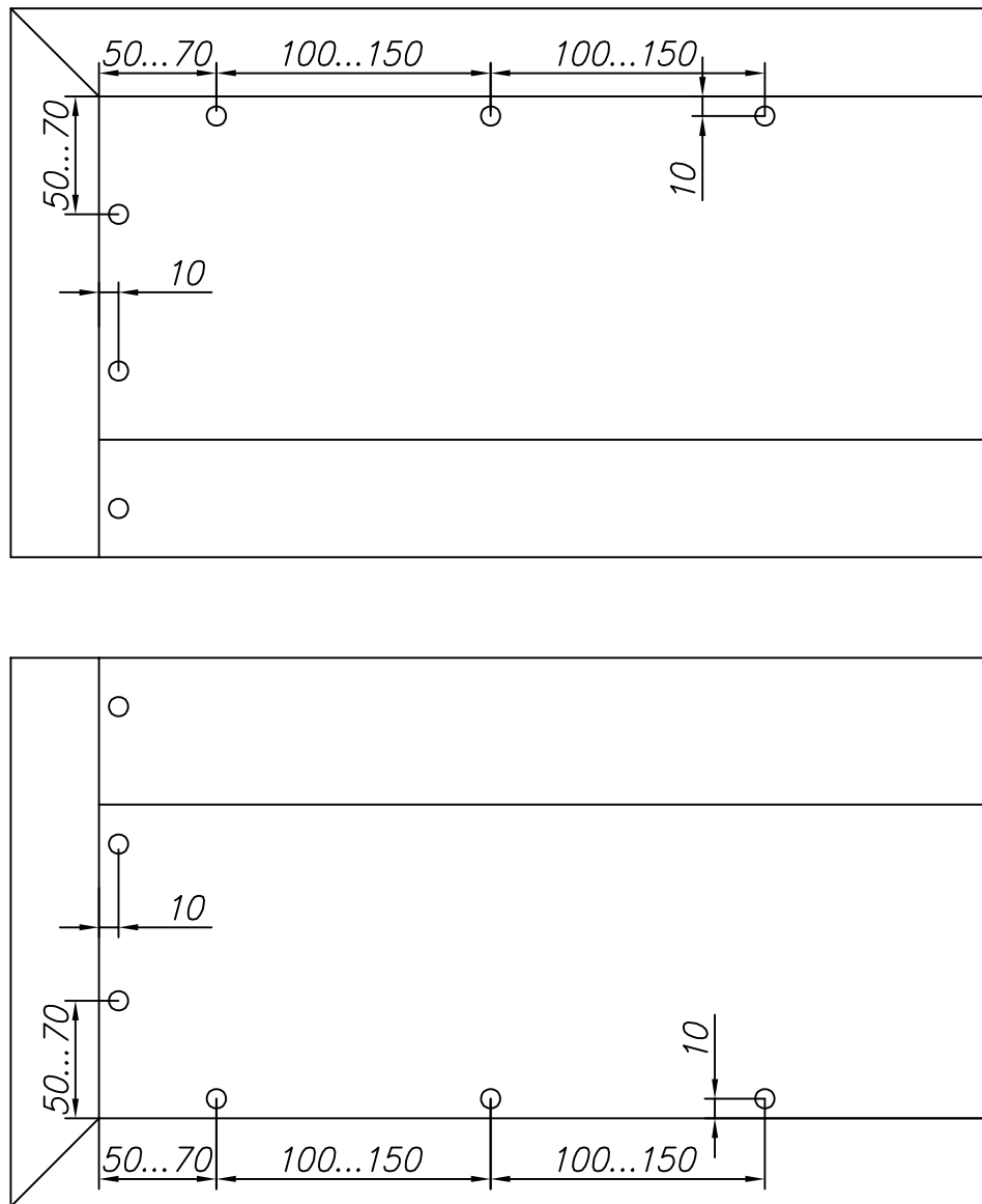
Рис. 8.26 – Разметка отверстий для установки винтов самонарезающих
