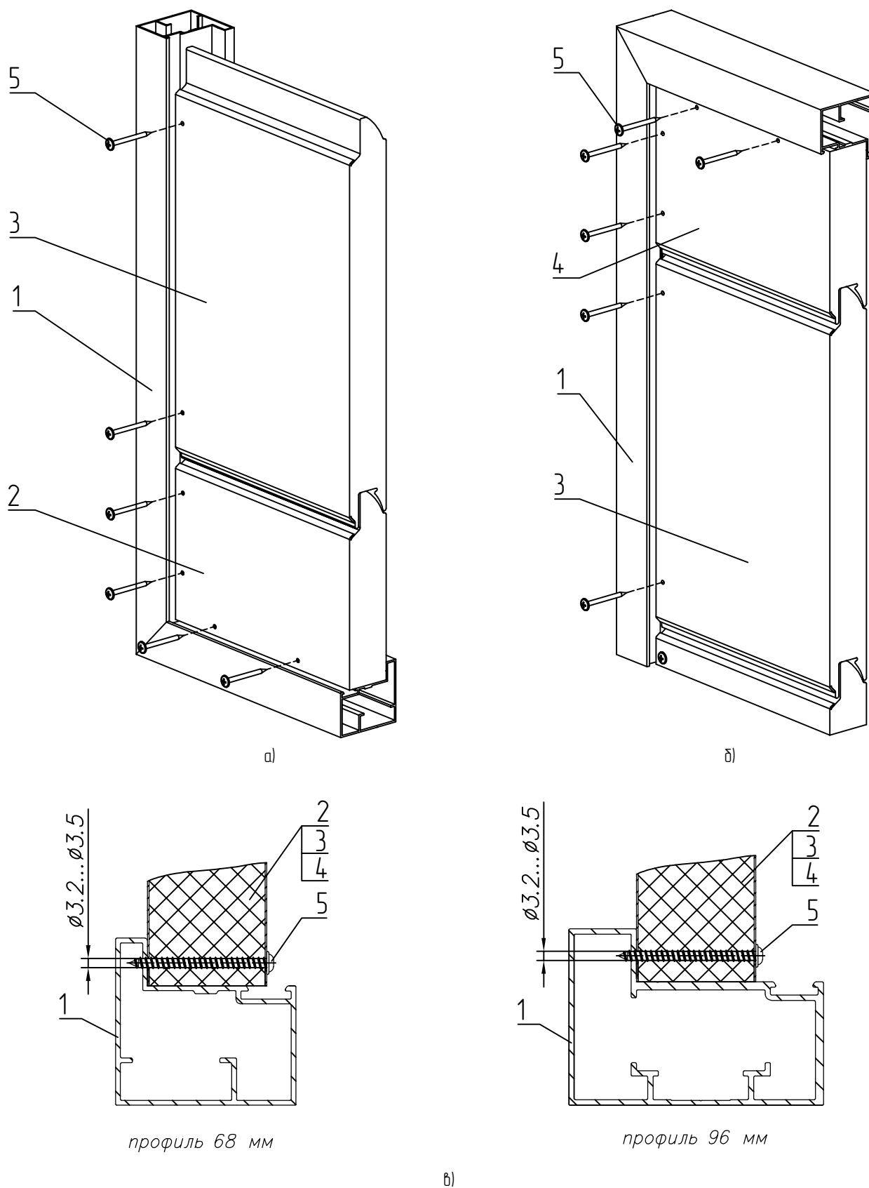
Рис. 8.27 – Закрепление сэндвич-панелей:
