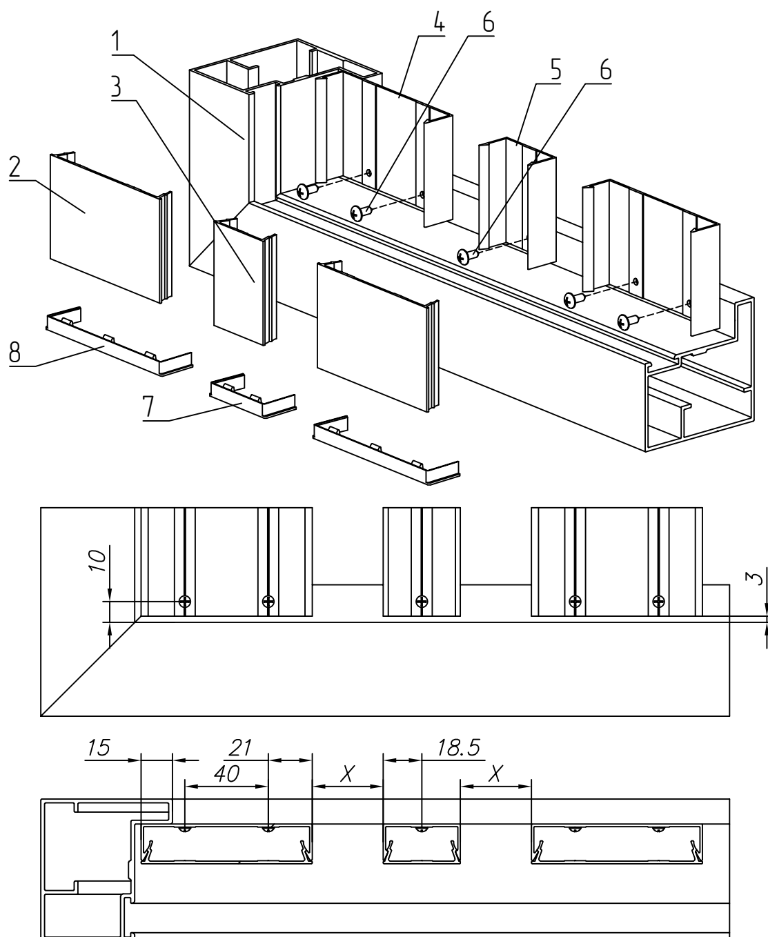
Рис. 8.4 – Монтаж разреженного заполнения со встроенным типом монтажа из сочетания профилей заполнения шириной 82 мм и 37 мм:
