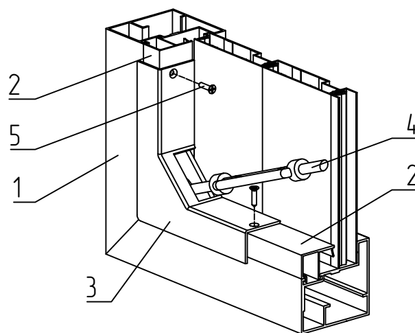
Рис. 9.5 – Установка крышки FLGU.400.0717:
