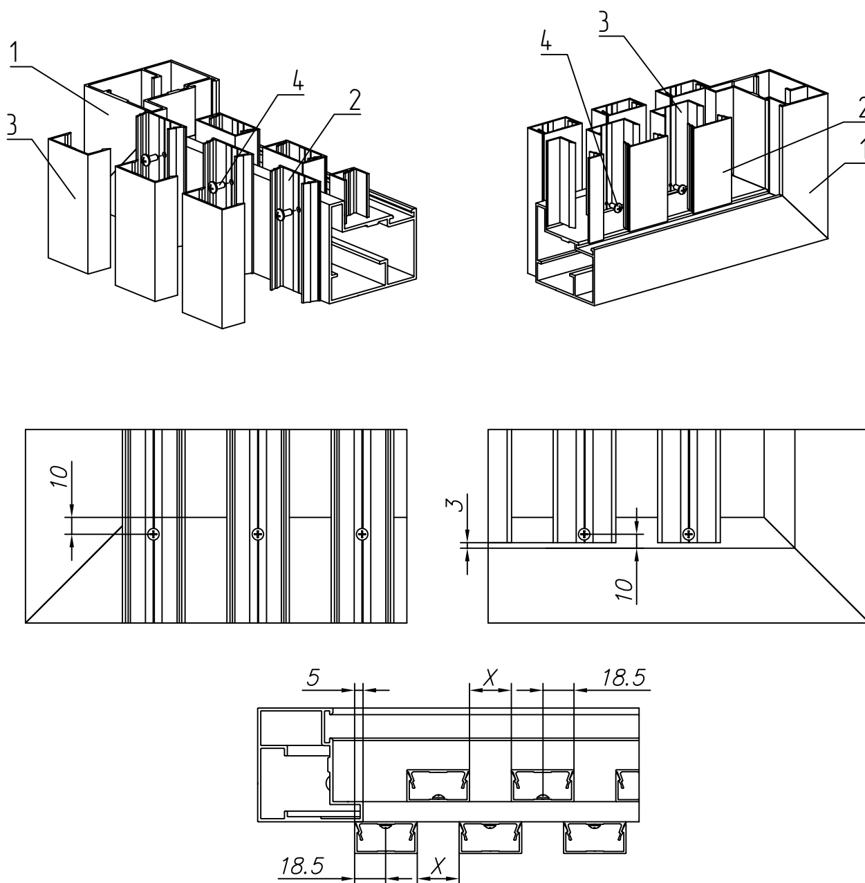
Рис. 8.17 – Шахматное заполнение из профилей шириной 37 мм:
