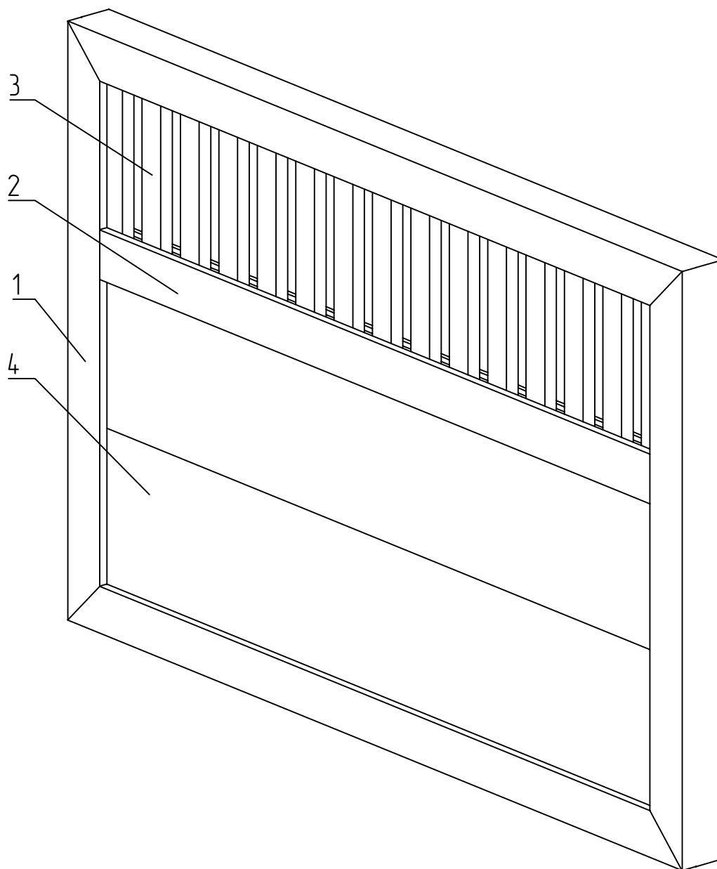
Рис. 8.35 – Створка с комбинированным заполнением: 1 – створка, 2 – разделительный импост, 3 – верхнее заполнение, 4 – нижнее заполнение
