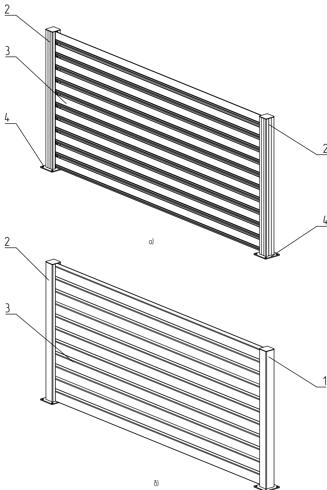
Рис. 7.7.7 – Секция заборная "Prestige Max" с заполнением алюминиевыми профилями (жалюзи): а) вид со стороны двора, б) вид со стороны улицы; 1 – столб угловой, 2 – столб прямой, 3 – заполнение, 4 – кронштейн для крепления секции
