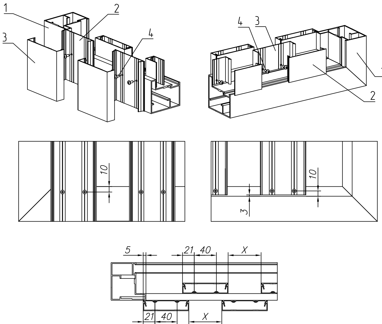
Рис. 8.16 – Шахматное заполнение из профилей шириной 82 мм: 1 – створка, 2 – профиль монтажный FLGU.400.0401, 3 – профиль разреженного заполнения FLGU.400.0403, 4 – винт самонарезающий 3,5х9,5SAX
