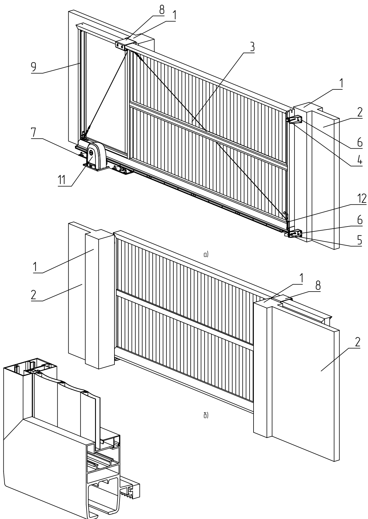
Рис. 7.17 – Откатные самонесущие ворота с вертикальным заполнением из профиля AG/77, открывание влево, без столбов удерживающих:
