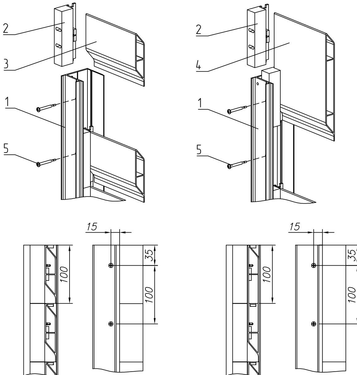
Рис. 8.23 – заполнение из алюминиевых профилей "жалюзи":
