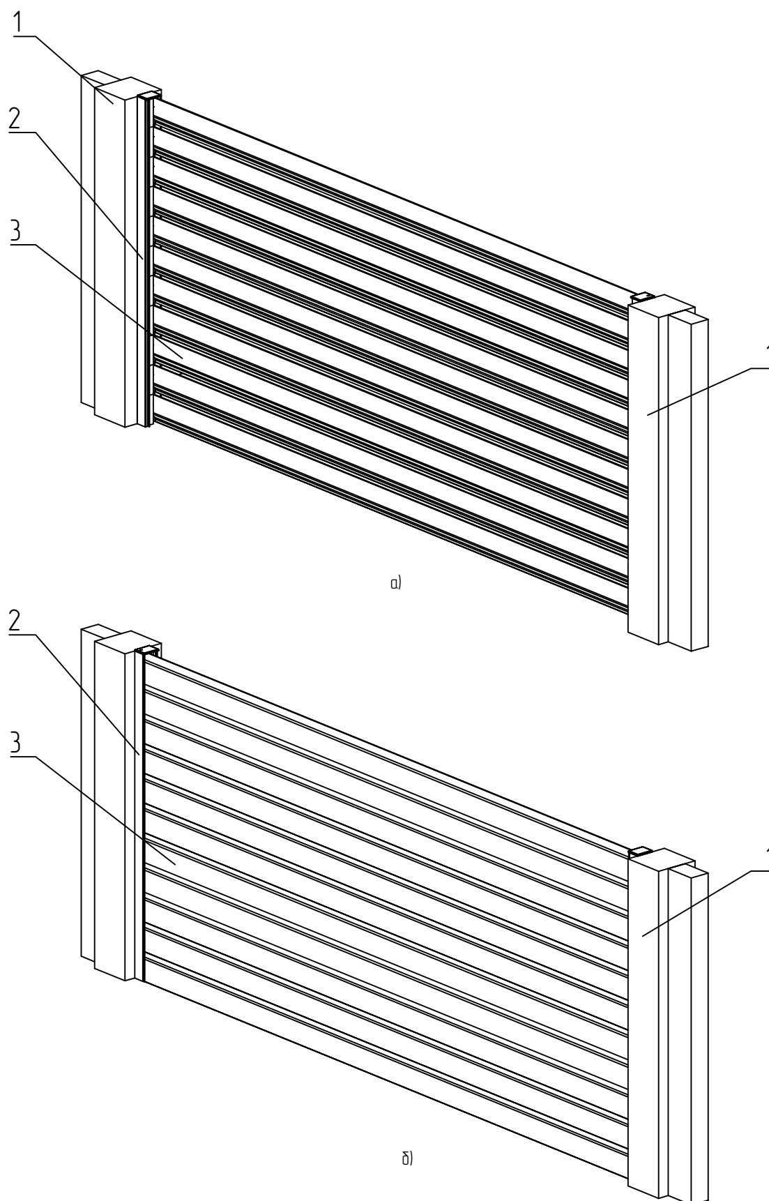
Рис. 7.7.6 – Секция заборная "Prestige Light" с заполнением алюминиевыми профилями (жалюзи): а) вид со стороны двора, б) вид со стороны улицы; 1 – столб проема, 2 – стойка секции, 3 – заполнение.
