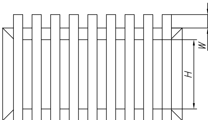
Рис. 8.36 – Размеры H и W при заполнении с накладным типом монтажа
