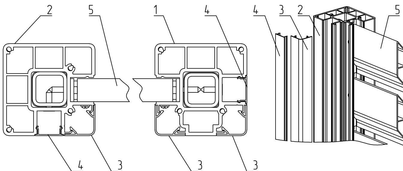
Рис. 9.9 – Установка штапиков 1 – столб (профиль FLGU.400.0507), 2 – столб (профиль FLGU.400.0508), 3 – штапик (профиль FLGU.400.0308), 4 – штапик (профиль FLGU.400.0309), 5 – заполнение.
