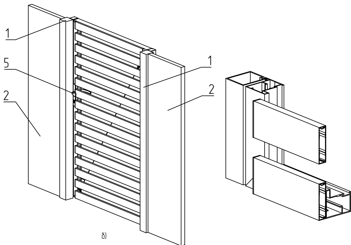
Рис. 7.6.3 – Калитка с накладным монтажом, направлением открывания влево, внутрь с горизонтальным накладным разрезным заполнением алюминиевыми профилями:
