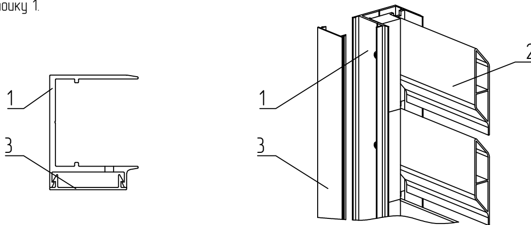
Рис. 9.8 – Установка штапика (профиль FLGU.400.0307) 1 – стойка (профиль FLGU.400.0119), 2 – заполнение, 3 – штапик.
