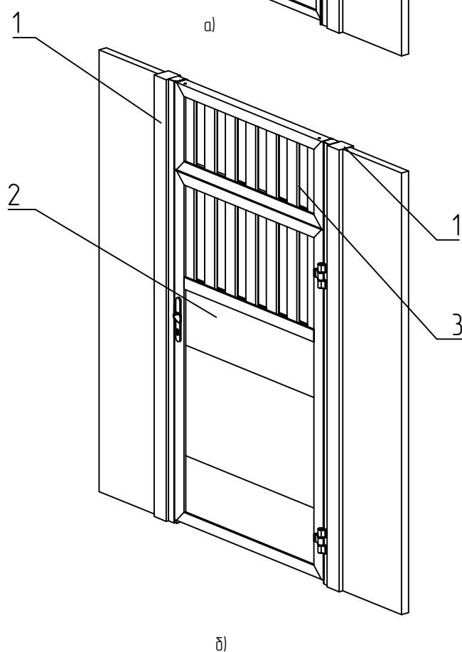
Рис. 7.7.3 – Фальш-панель с вертикальным встроенным разреженным заполнением алюминиевыми профилями над калиткой со встроенным монтажом, направлением открывания вправо, наружу: а) вид со стороны двора, б) вид со стороны улицы; 1 – столб проема, 2 – калитка, 3 – фальш-панель
