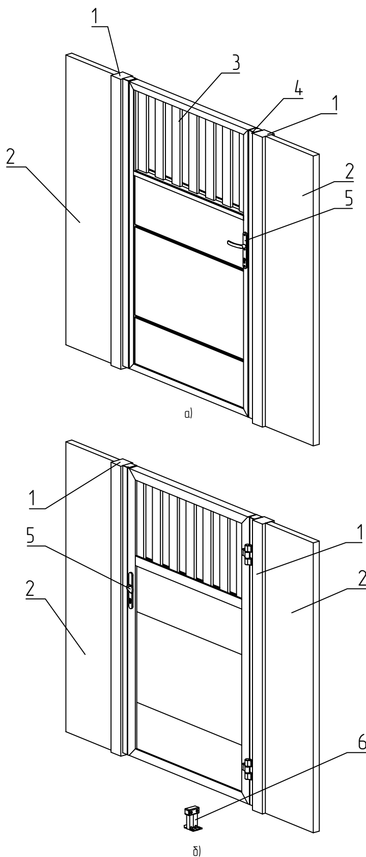
Рис. 7.6.6 – Калитка со встроенным монтажем, направлением открывания вправо, наружу с комбинированным заполнением из сэндвич-панели и алюминиевого профиля:
