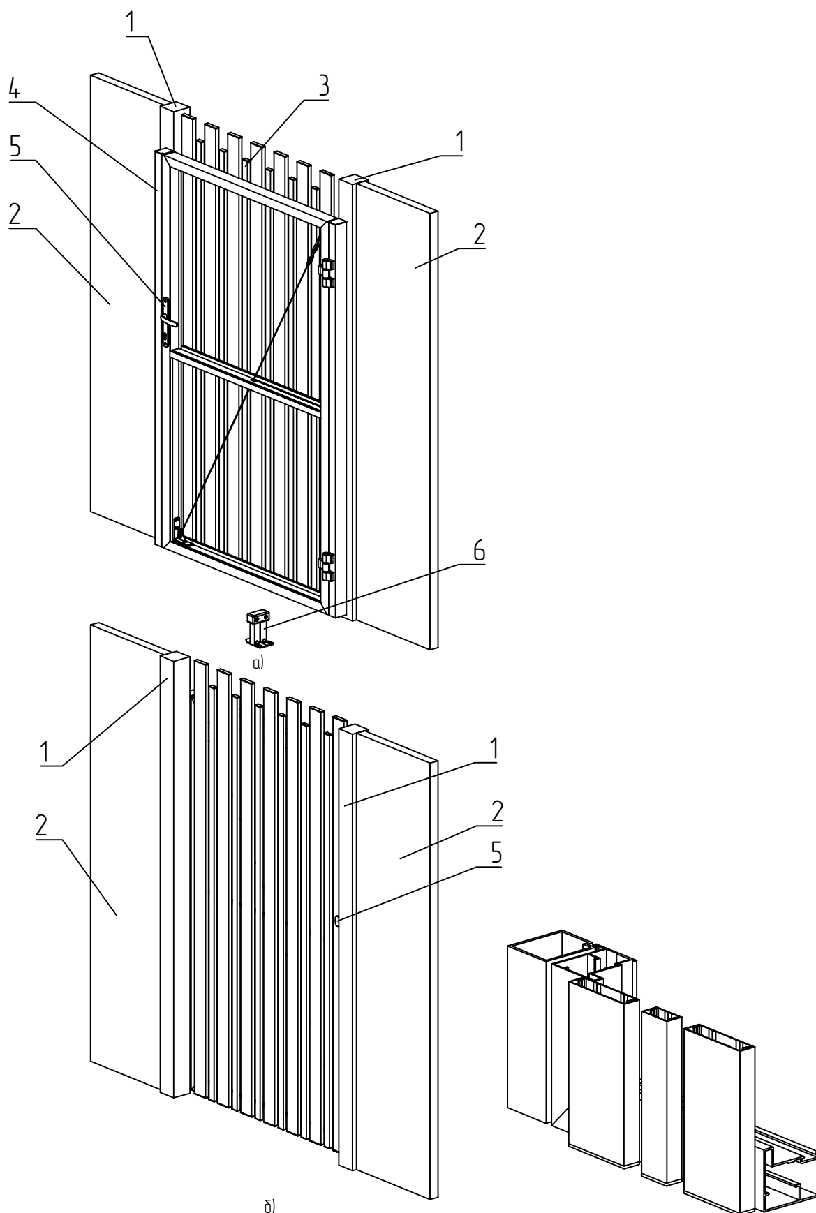
Рис. 7.6.4 – Калитка с накладным монтажом, направлением открывания вправо, внутрь с вертикальным накладным разреженным заполнением алюминиевыми профилями (гребенка):
