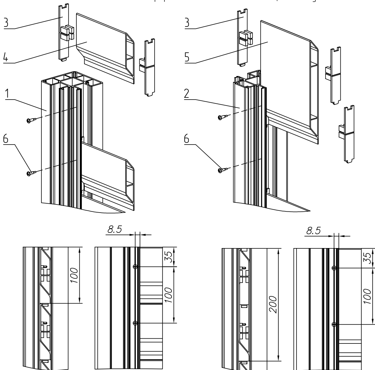
Рис. 8.22 – заполнение из алюминиевых профилей "жалюзи":
