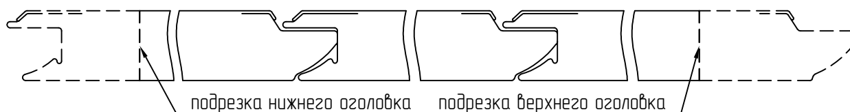
Рис. 8.24 – Заполнение из сэндвич-панели
