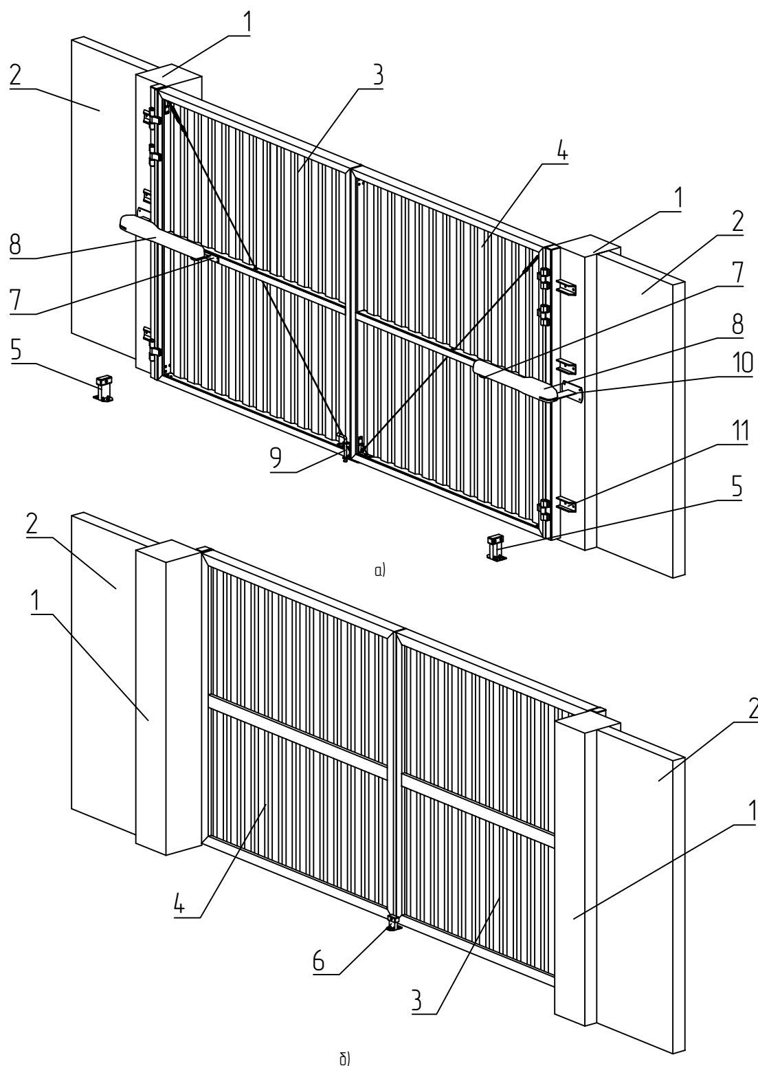
Рис. 7.4.2 – Распашные ворота с накладным типом монтажа, открывание внутрь со встроенным заполнением из профилированного листа: а) вид со стороны двора, б) вид со стороны улицы;
