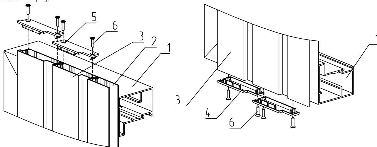
Рис. 8.15 – Установка крышек:
